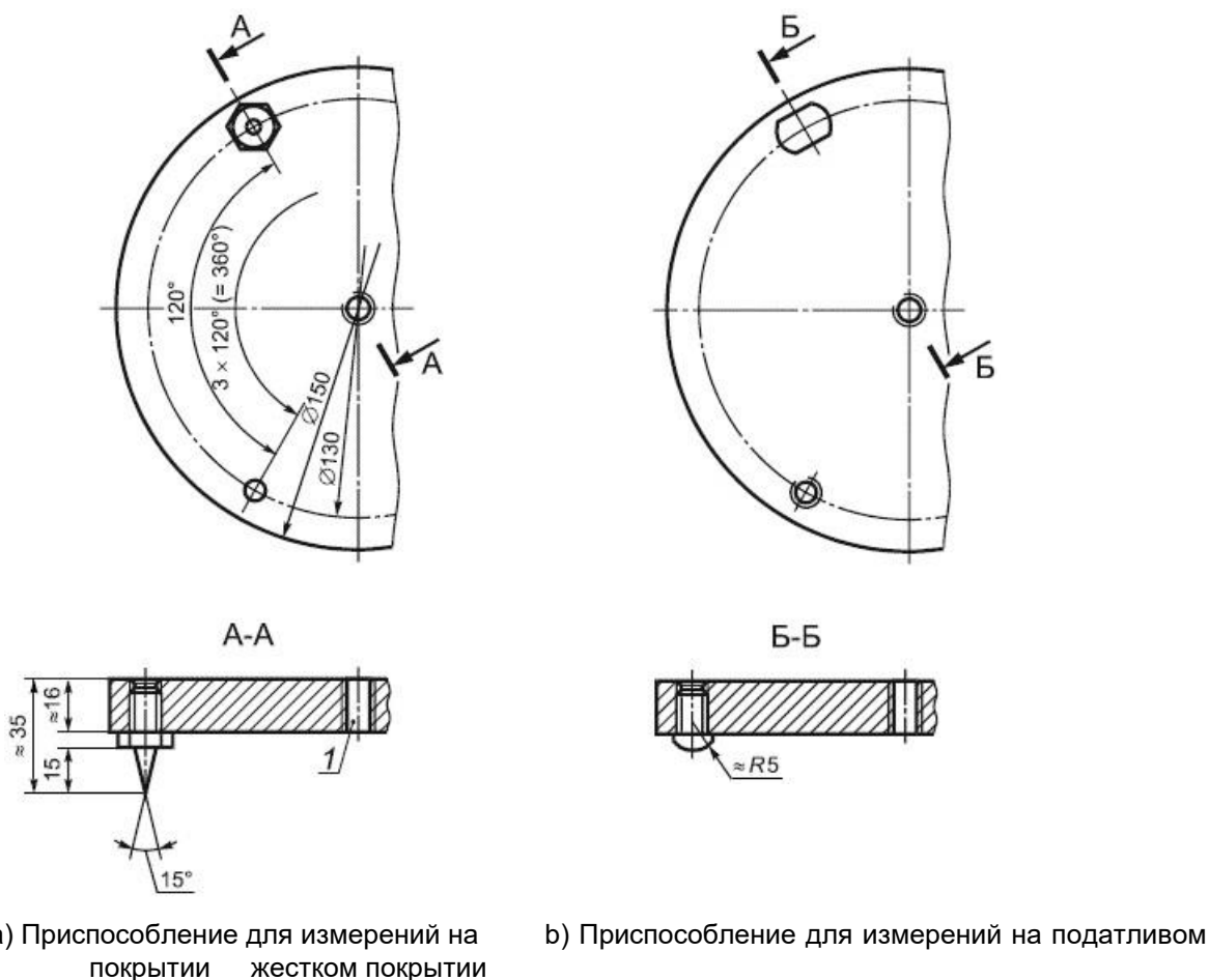
Рисунок 1 - Приспособления для быстрой установки датчиков вибрации
